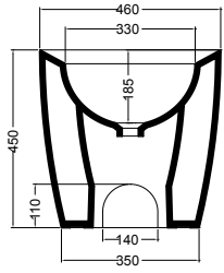
SEZIONE LONGITUDINALE LONGITUDINAL VIEW
